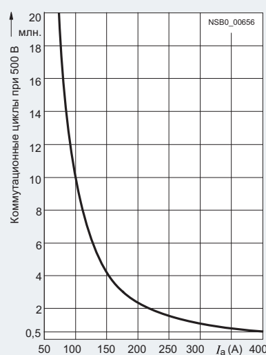
Контакторы ЗТС74 - ЗТС78
